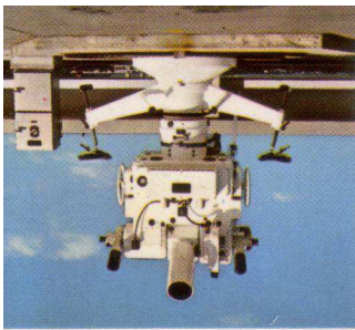
Flugbahnvermessungsanlage EOTS
